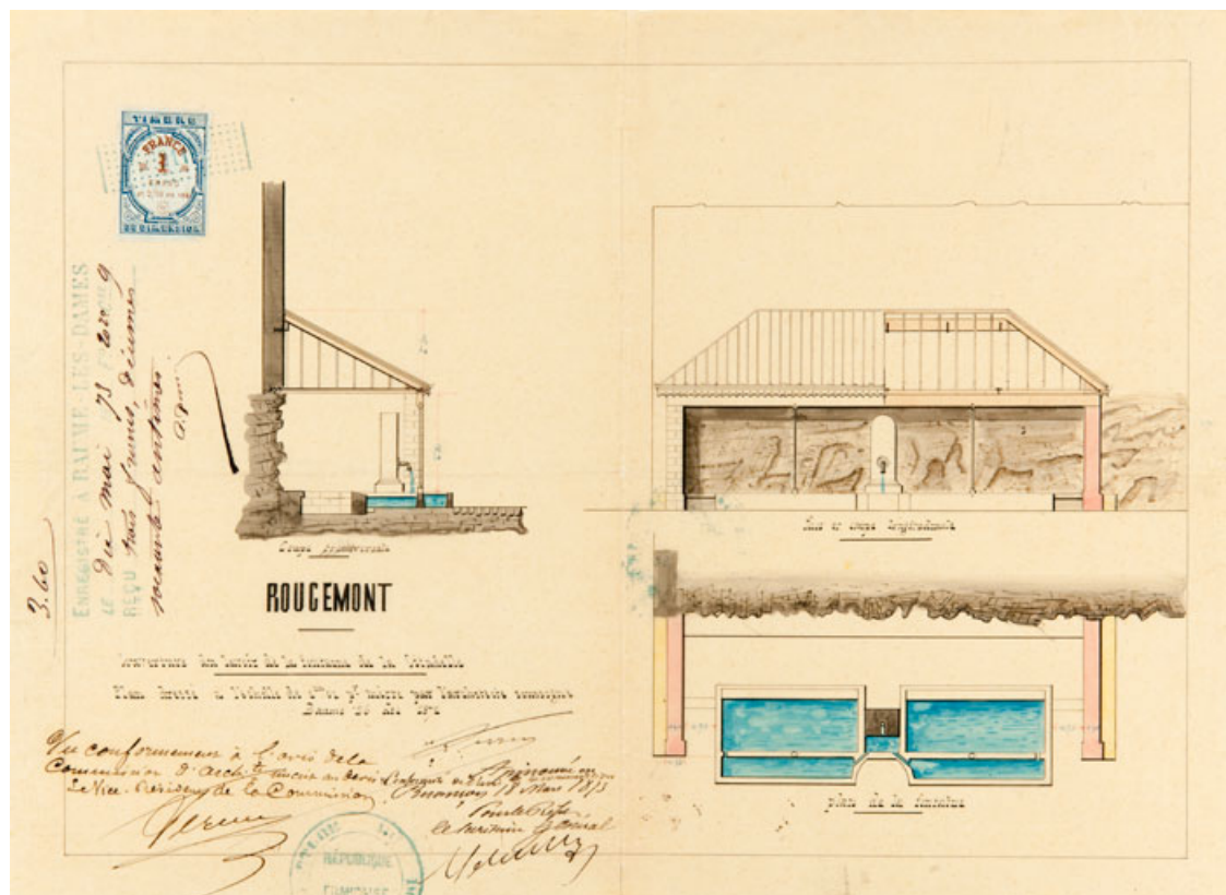
Rougemont. Couverture du lavoir de la fontaine de la Citadelle. Coupe transversale. Face et coupe longitudinale. Plan de la fontaine.
