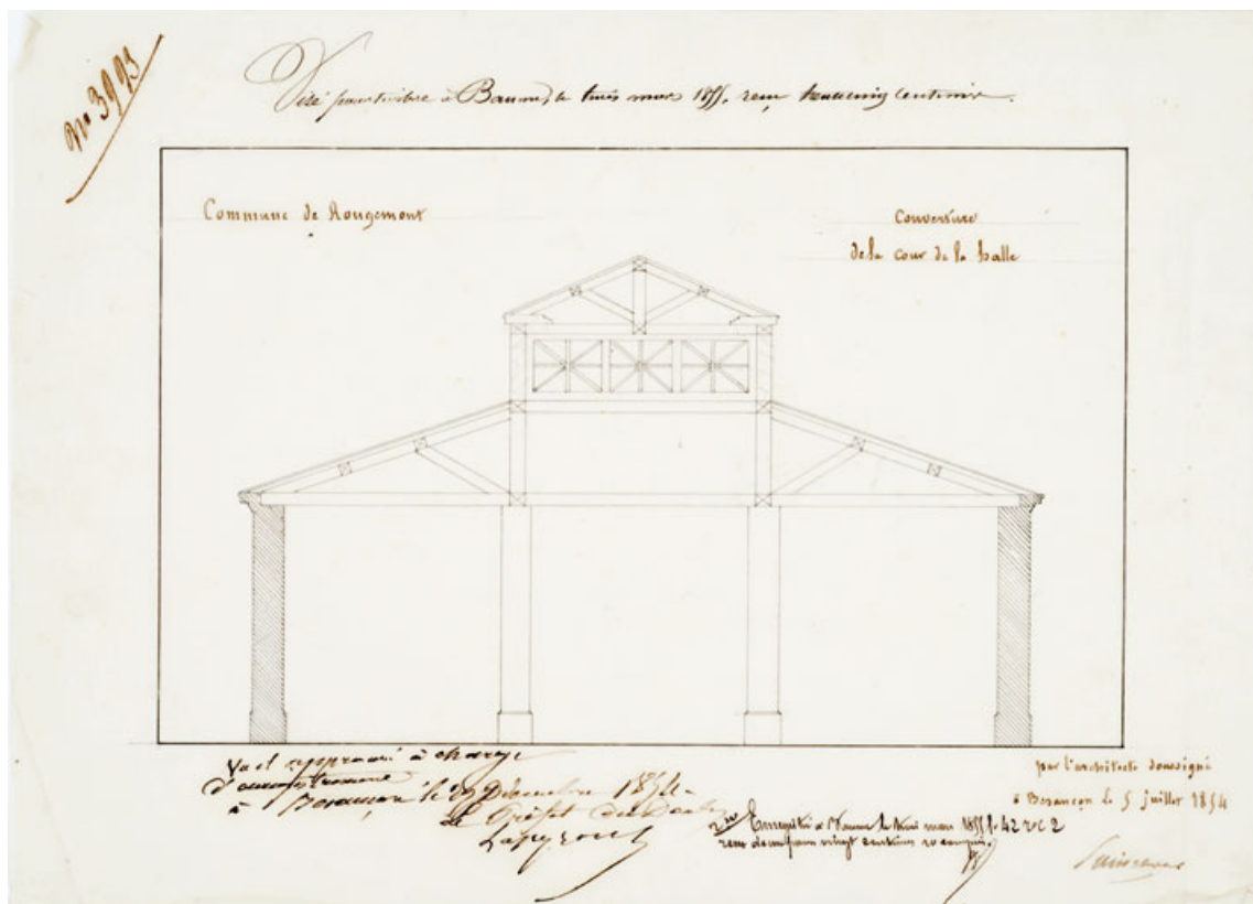
Commune de Rougemont. Couverture de la cour de la halle. 25, Rougemont rue du Lavoir
