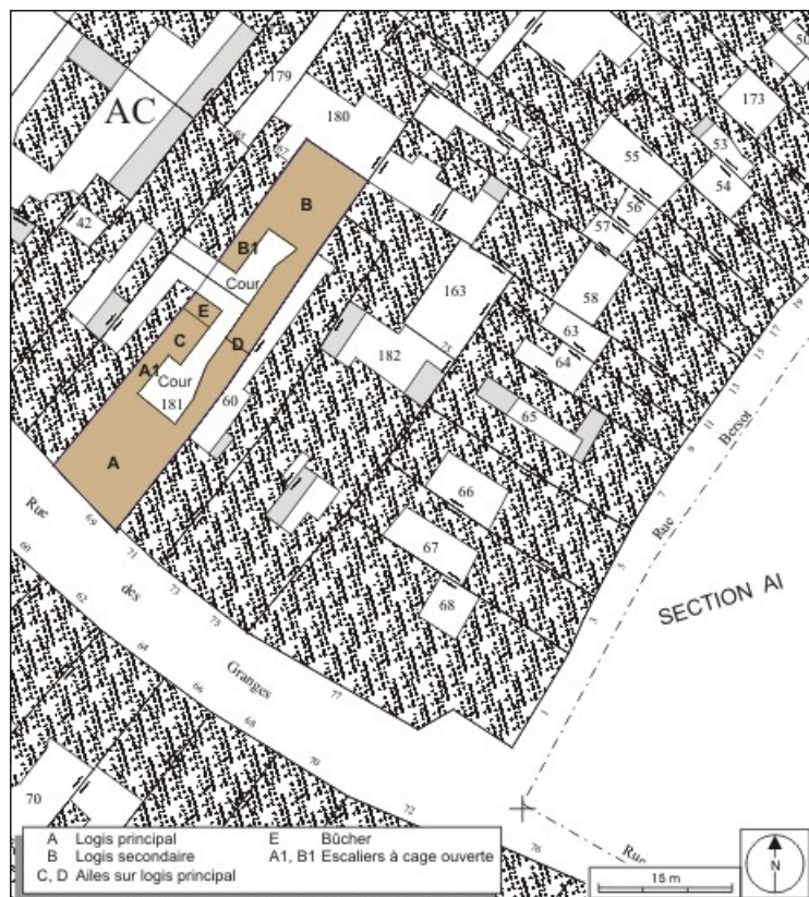
Plan masse et de situation. Extrait du plan cadastral, 1974, section AC. 25, Besançon, 69 rue des Granges, lieudit : îlot Proudhon
