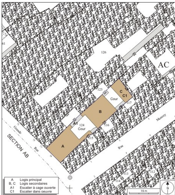
Plan masse et de situation. Extrait du plan cadastral, 1974, section AC. 25, Besançon Grande Rue 79, lieudit : îlot Saint-Pierre
