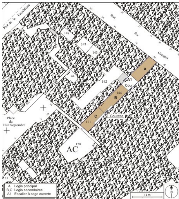
Plan masse et de situation. Extrait du plan cadastral, 1974, section AC. 25, Besançon, 40 rue des Granges, lieudit : îlot Saint-Pierre
