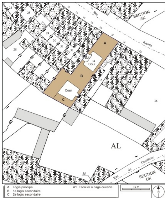
Plan masse et de situation. Extrait du plan cadastral, 1974, section AL. 25, Besançon, 22 rue Rivotte, lieudit : îlot Boitouset
