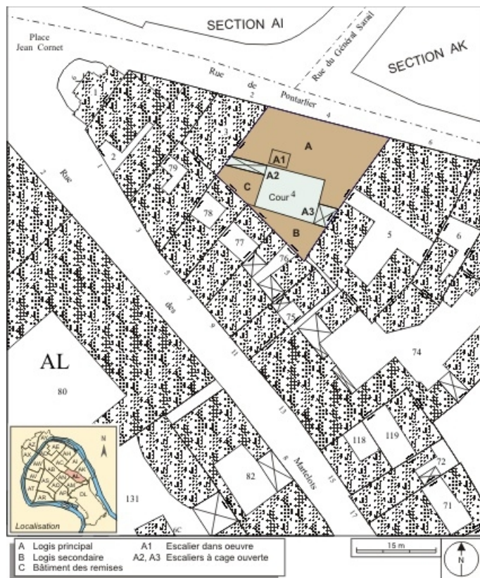
Plan masse et de situation. Extrait du plan cadastral, 1974, section AL. 25, Besançon, 4 rue de Pontarlier, lieudit : îlot des Martelots
