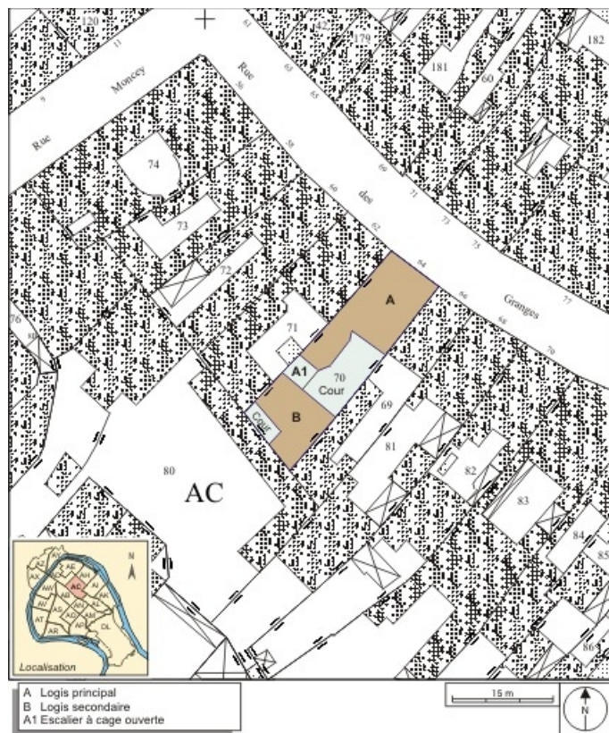
Plan masse et de situation. Extrait du plan cadastral, 1974, section AC. 25, Besançon, 64 rue des Granges, lieudit : îlot Forum
