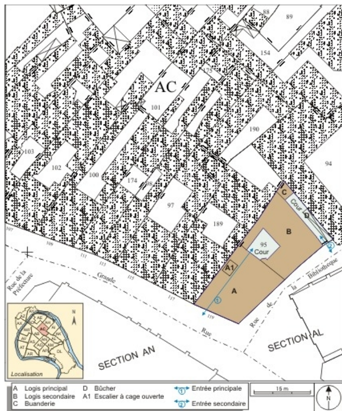
Plan masse et de situation. Extrait du plan cadastral, 1974, section AC. 25, Besançon Grande Rue 119, lieudit : îlot Forum
