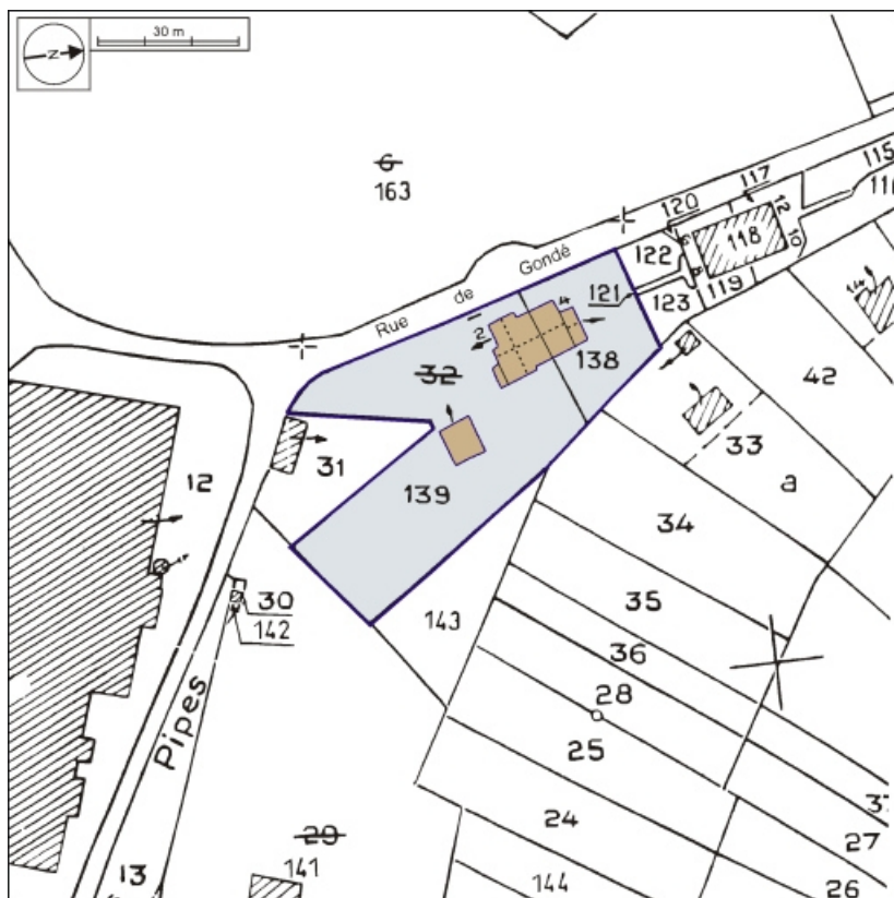
Plan-masse et de situation. Extrait du plan cadastral, 1982, section ZN, 1:2000 agrandi à 1:1000. 25, Baume-les-Dames, 2, 4 rue de Gondé, lieudit : Gondé
