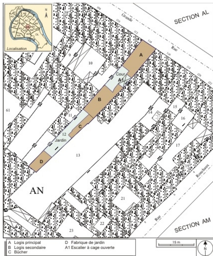
Plan masse et de situation. Extrait du plan cadastral, 1974, section AN. 25, Besançon Grande Rue 114, lieudit : îlot Granvelle
