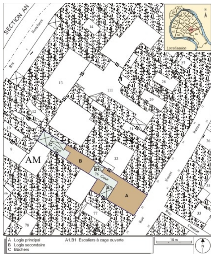
Plan masse et de situation. Extrait du plan cadastral, 1974, section AM. 25, Besançon, 22 rue Renan, lieudit : îlot Ronchaux
