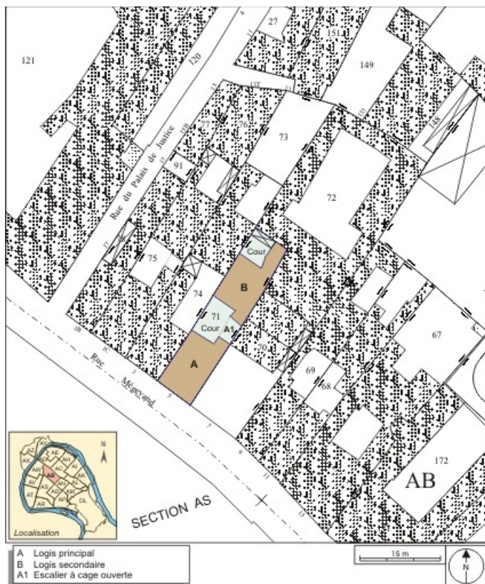
Plan masse et de situation. Extrait du plan cadastral, 1974, section AB. 25, Besançon, 5 rue Mégevand, lieudit : îlot Terrier de Santans
