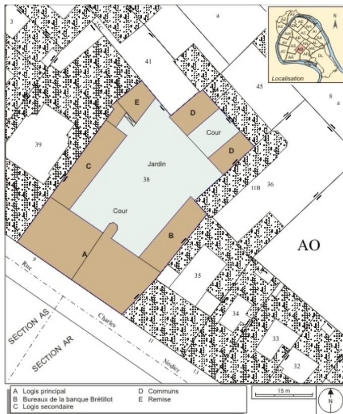
Plan masse et de situation. Extrait du plan cadastral, 1993, section AO. 25, Besançon, 9, 9 bis rue Charles Nodier, lieudit : îlot Banque de France
