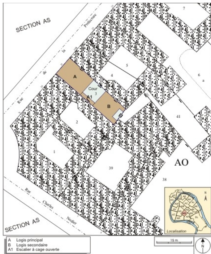
Plan masse et de situation. Extrait du plan cadastral, 1993, section AO. 25, Besançon, 27 rue de la Préfecture, lieudit : îlot Banque de France
