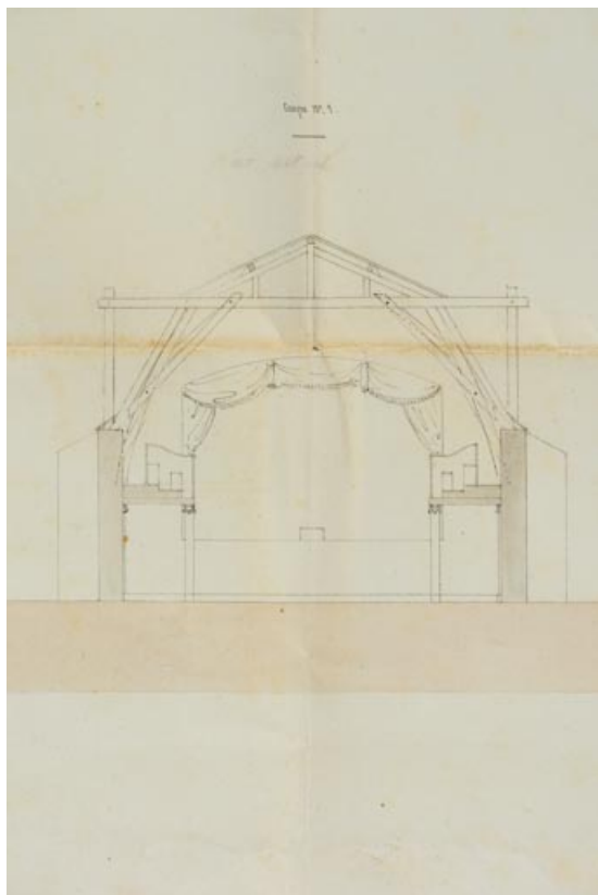
Ville d'Auxonne. Projets de réparations à la salle de spectacle. [Détail de la coupe transversale : avant transformation]. 3 mai 1842. 21, Auxonne boulevard Pasteur
