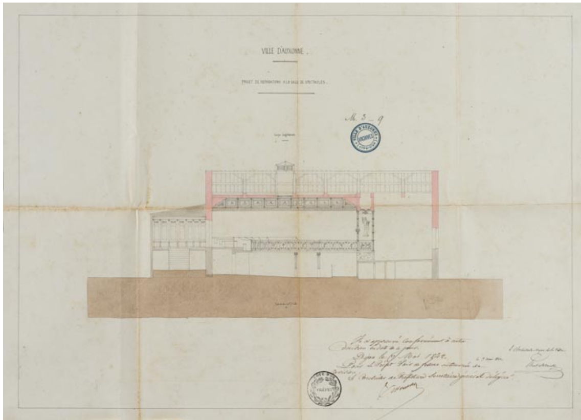
Ville d'Auxonne. Projets de réparations à la salle de spectacle. [Coupe longitudinale]. 3 mai 1842. 21, Auxonne boulevard Pasteur
