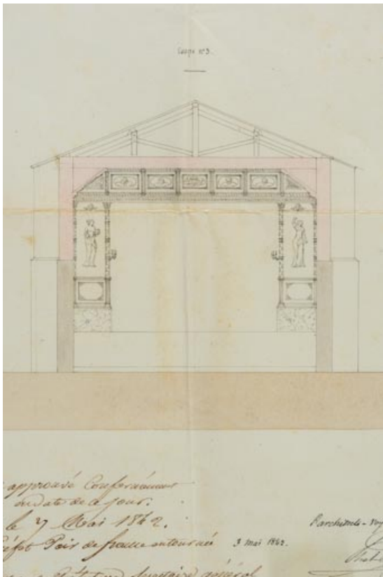
Ville d'Auxonne. Projets de réparations à la salle de spectacle. [Détail de la coupe transversale : côté scène]. 3 mai 1842. 21, Auxonne boulevard Pasteur
