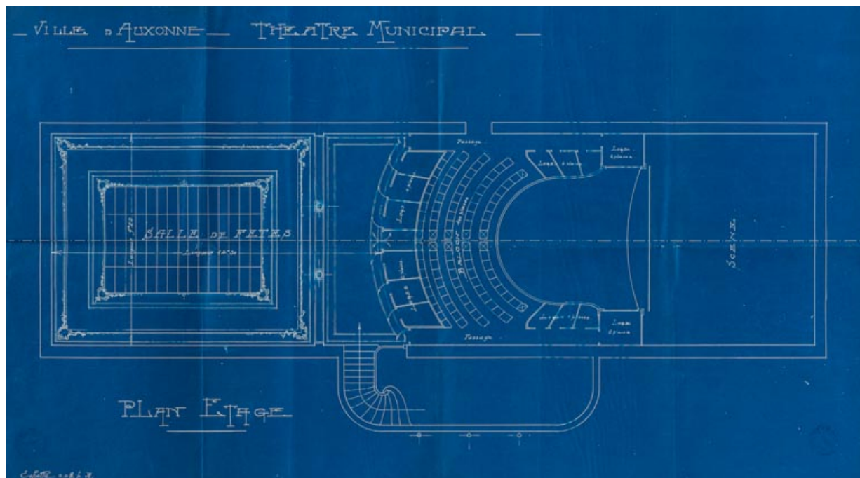
Ville d'Auxonne. Théâtre municipal. Plan étage.
