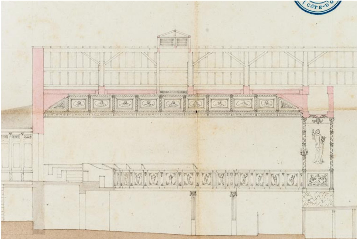
Ville d'Auxonne. Projets de réparations à la salle de spectacle. [Détail de la coupe longitudinale]. 3 mai 1842. 21, Auxonne boulevard Pasteur
