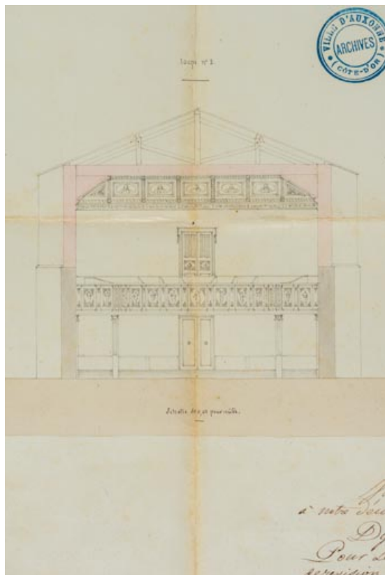
Ville d'Auxonne. Projets de réparations à la salle de spectacle. [Détail de la coupe transversale : côté entrée]. 3 mai 1842. 21, Auxonne boulevard Pasteur
