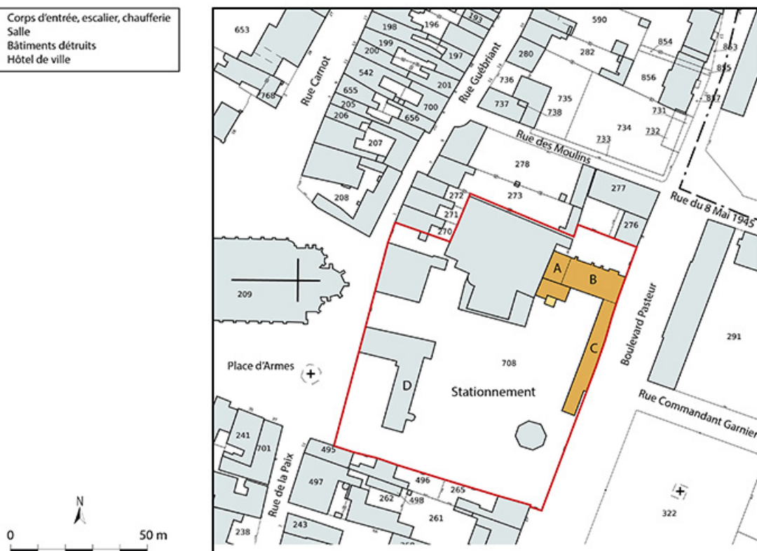
Plan-masse et de situation. Extrait du plan cadastral, 2021, section BL, 1/1 000. 21, Auxonne boulevard Pasteur
