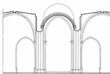
COUPE A.A'
