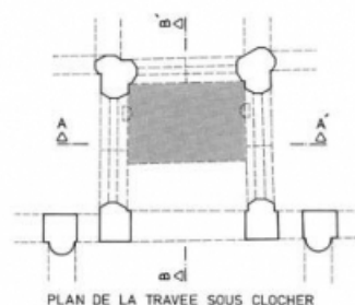
PLAN DE LA TRAVEE SOUS CLOCHER
