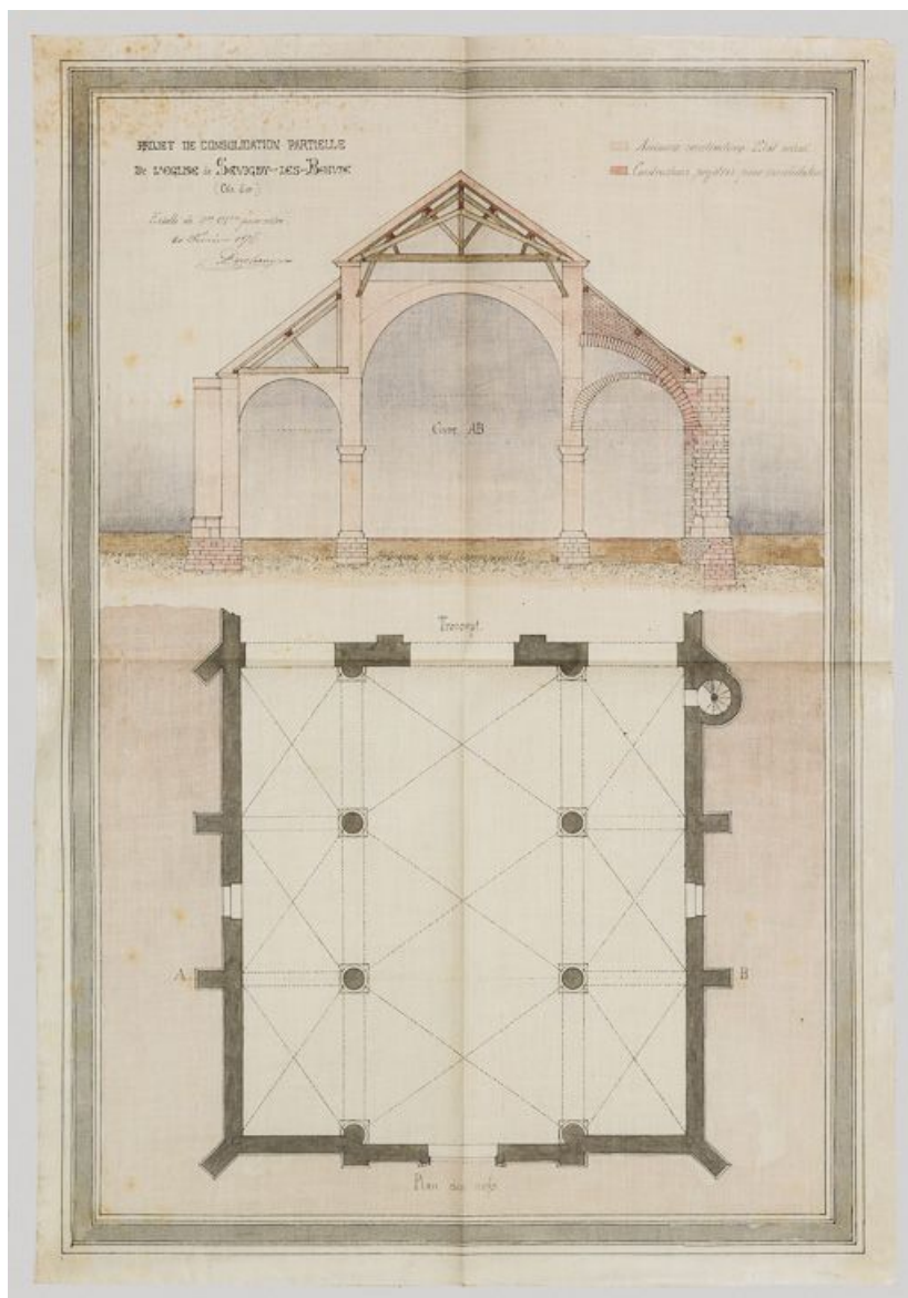
Projet de consolidation partielle de l'église de Savigny-lès-Beaune (Côte-d'Or)" : coupe et plan. Daté du 20 février 1874 et signé Deschamp. (Archives municipales, Savigny-lès-Beaune) 21, Savigny-lès-Beaune place de l' Eglise
