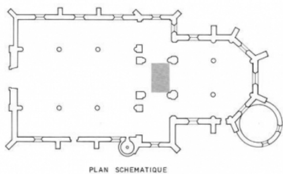
PLAN SCHEMATIQUE
