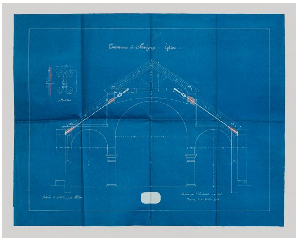
Coupe du projet de consolidation de l'église de Savigny-lès-Beaune. 6 juillet 1908. (Archives municipales, Savigny-lès-Beaune) 21, Savigny-lès-Beaune place de l' Eglise
