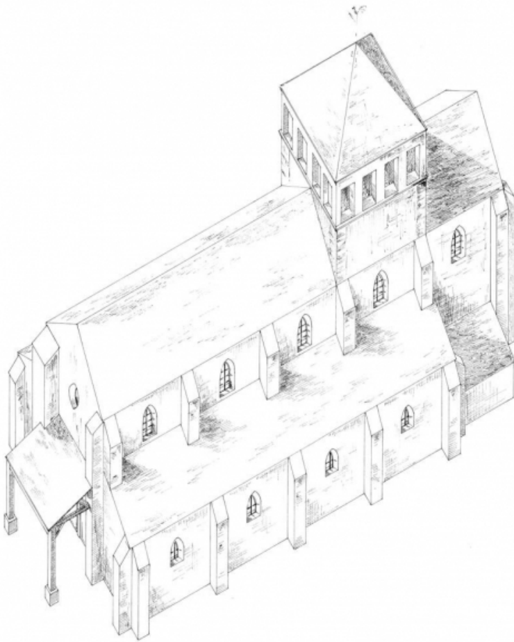
Vue axonométrique de l'ancienne église, reconstitution.
