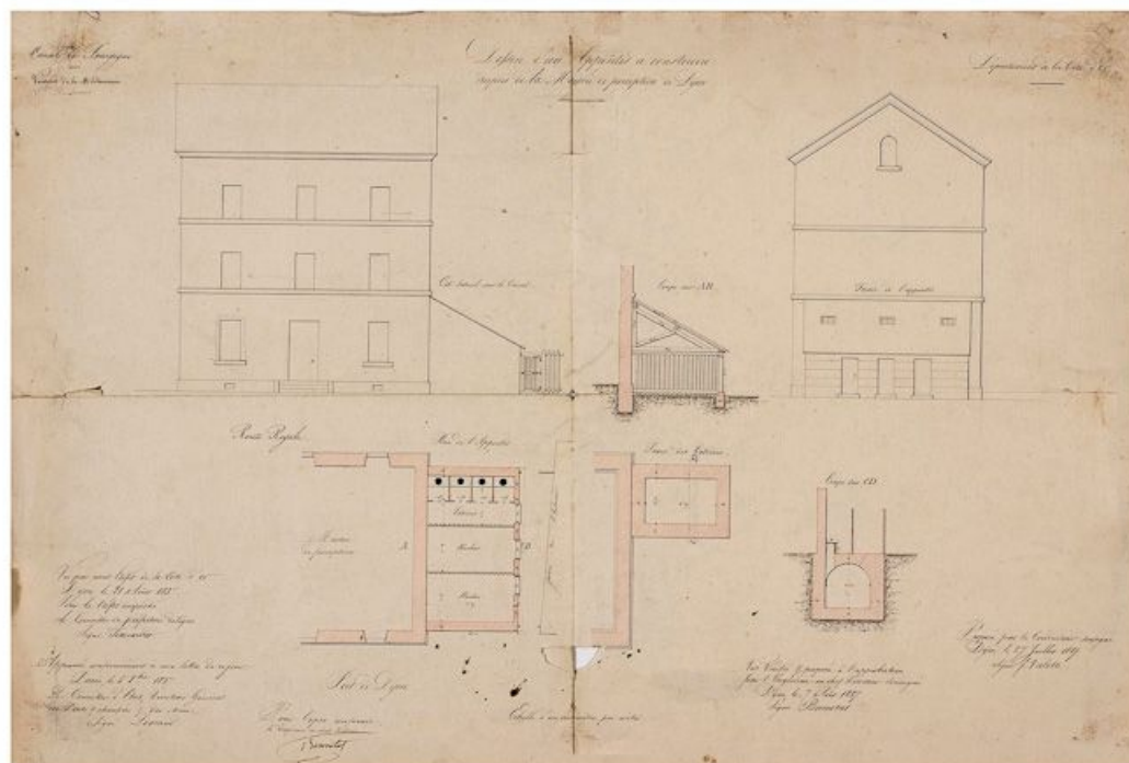
"Dessin d'un appentis à construire auprès de la maison de perception de Dijon". Plans, coupes et élévations. 1837. (Archives départementales de la Côte-d'Or, Dijon)
