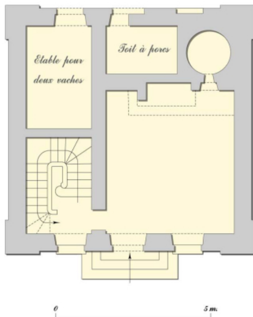
Maison d'éclusier par l'ingénieur Perronet, d'après un document ancien, plan du rez-de-chaussée.
