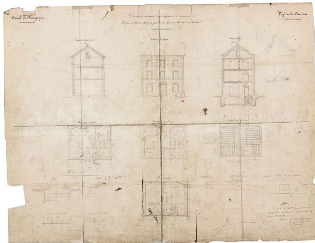
"Dessins des maisons de perception à construire à Dijon à Pont-de-Pany au port de la Maison-Blanche et à Montbard". 1836. (Archives départementales de la Côte-d'Or, Dijon)
