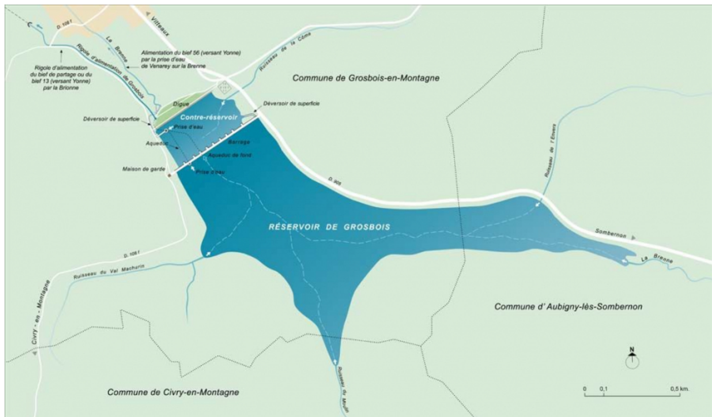
Plan schématique d'ensemble du réservoir de Grosbois.
