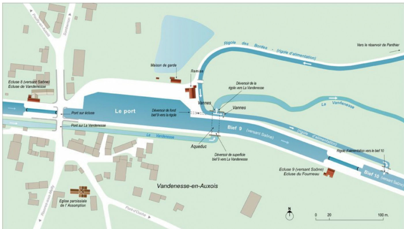
Plan schématique du port et du réseau hydraulique.
