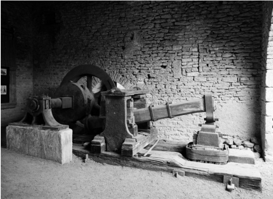
Forge d'affinerie, halle d'entrée, martinet de platinerie.
