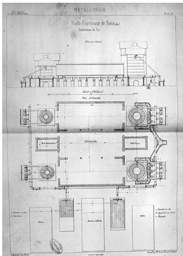
Hauts-Fourneaux de Rans (Jura). Distribution du gaz. 39, Rans
