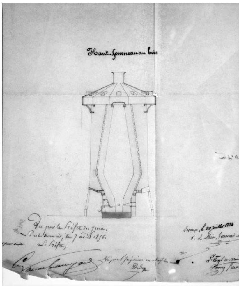
Coupe d'un haut-fourneau au bois.
