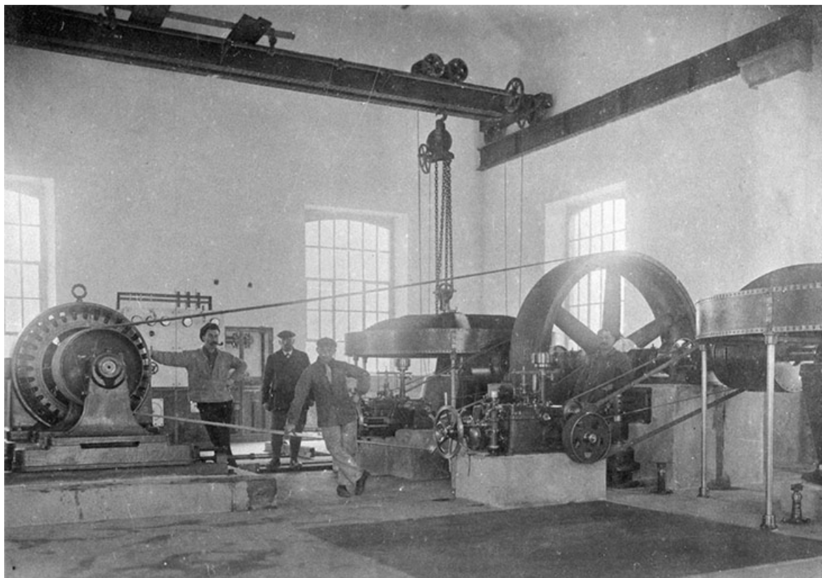
Intérieur de la centrale hydroélectrique.
