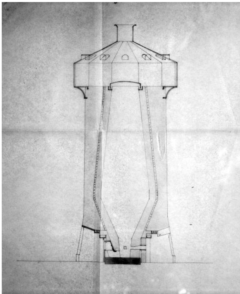
Coupe d'un haut-fourneau au coke.
