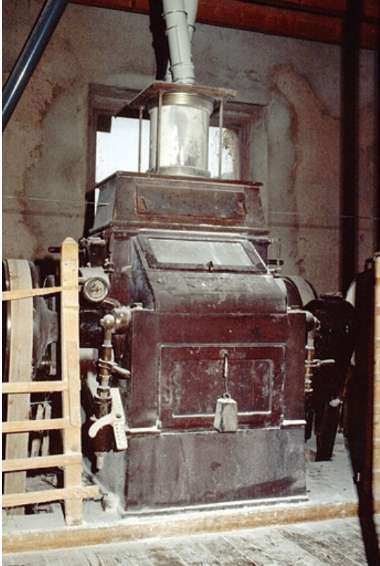
Minoterie (H), rez-de-chaussée : appareil à cylindres (convertisseur) Teisset-Rose-Brault. 39, Vaudrey rue du Moulin
