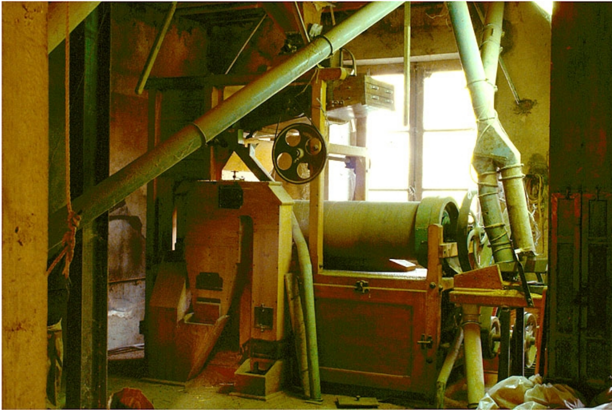
Minoterie (H), rez-de-chaussée : trieur à grains Lhuillier.
