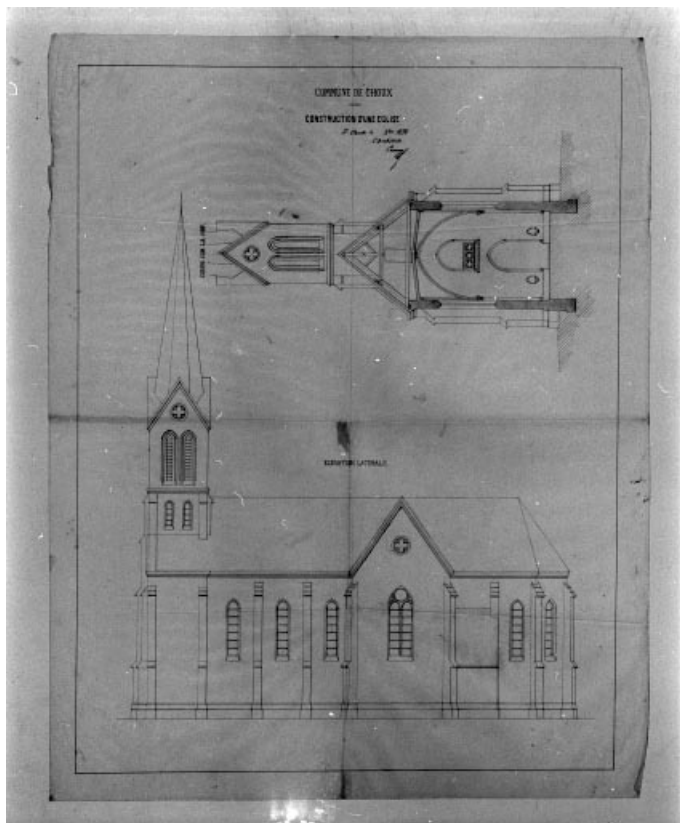
Commune de Choux. Construction d'une église [coupe sur la nef et élévation latérale].
