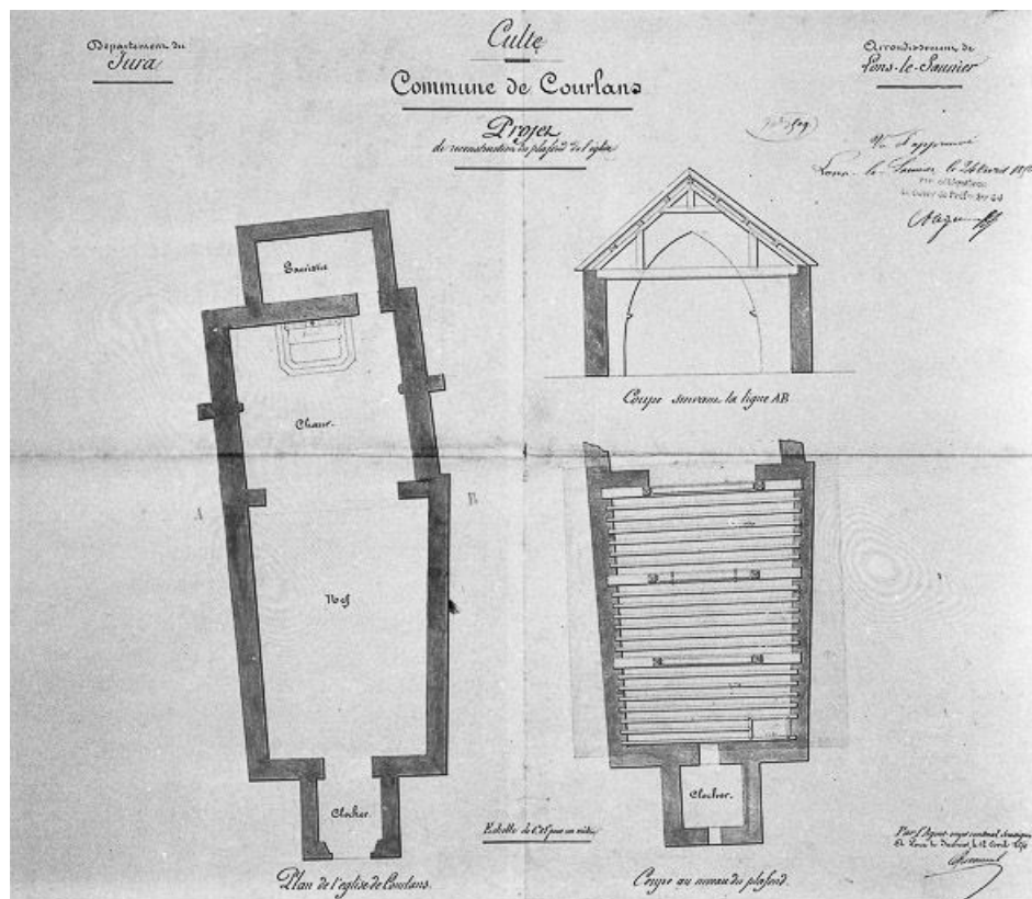
Plan, coupe transversale, coupe au niveau du plafond.
