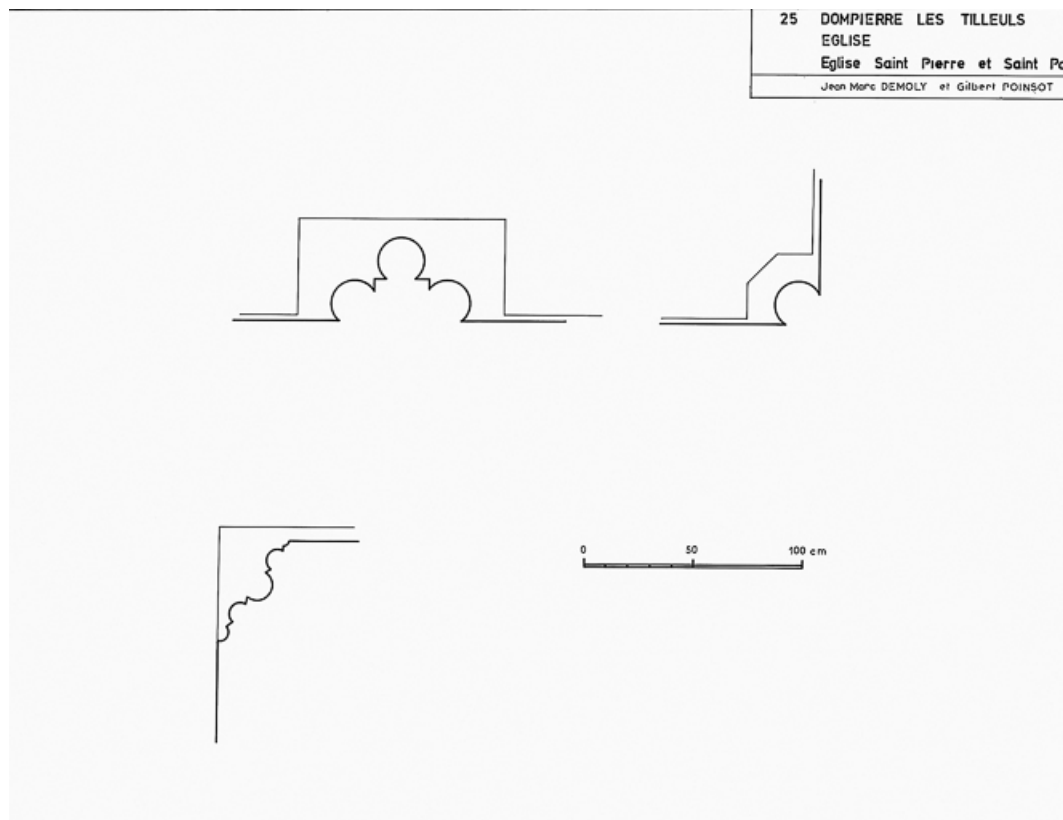
Détail : coupe des colonnes par J.-M. Demoly et Gilbert Poinso, 1975.
