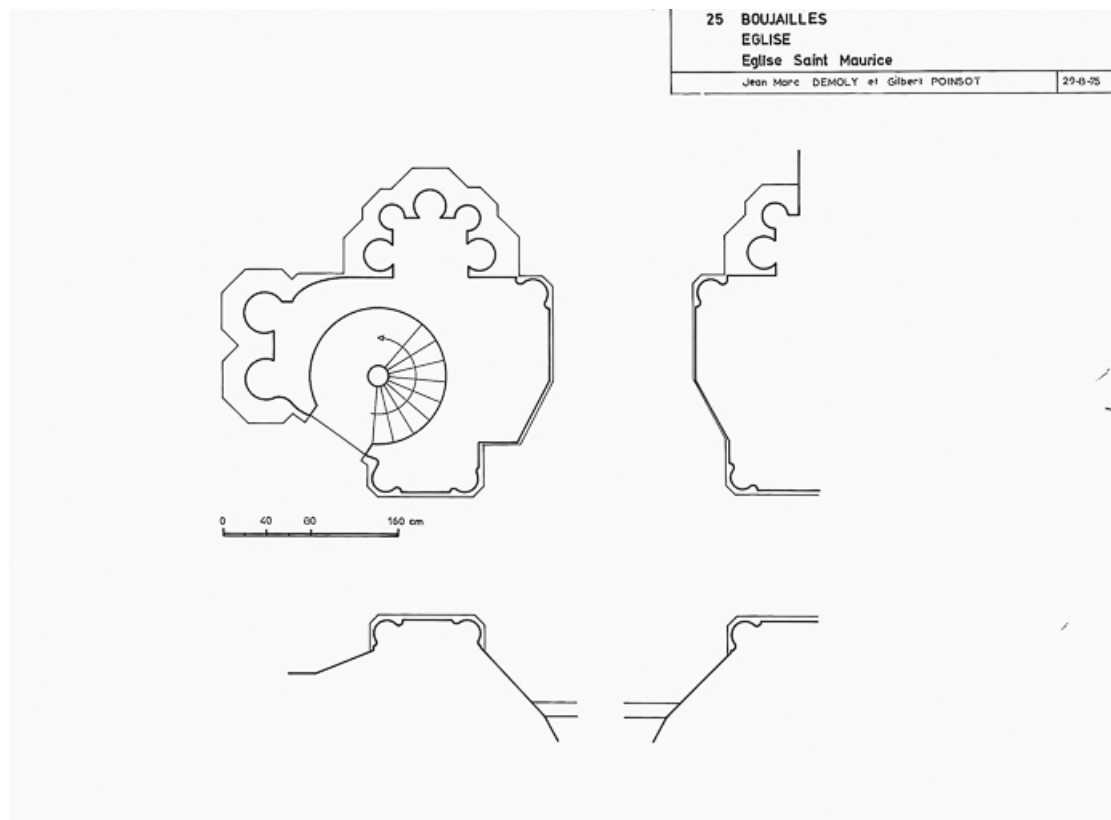
Plan des piliers d'entrée : relevé-croquis J.-M Demoly et Gilbert Poinsoy, 1975.
