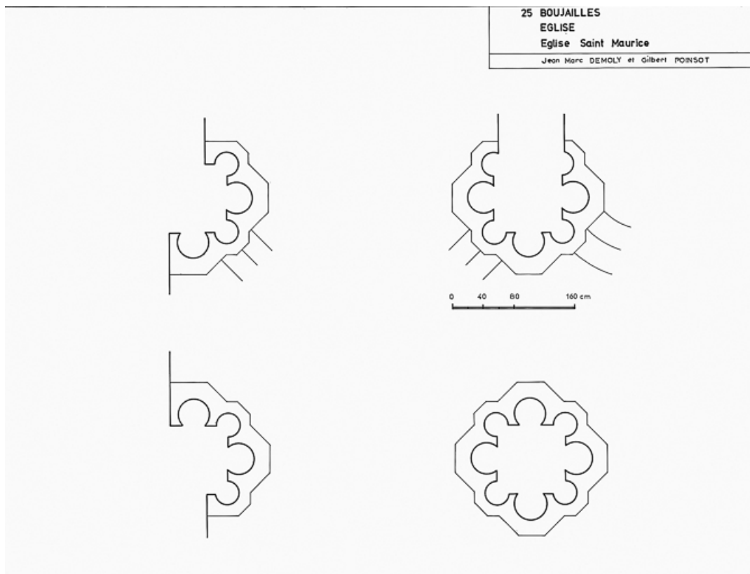
Plan des gros piliers : relevé-croquis J.-M Demoly et Gilbert Poinsoy, 1975.t, 1975.
