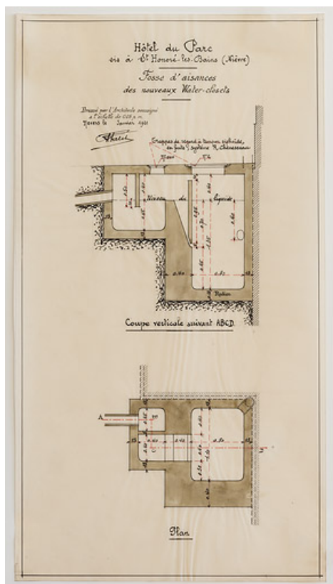
Fosse d'aisances, plan et coupe.
