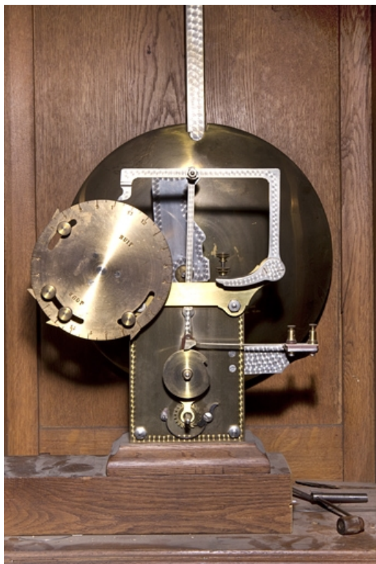
Système de programmation des sonneries.
