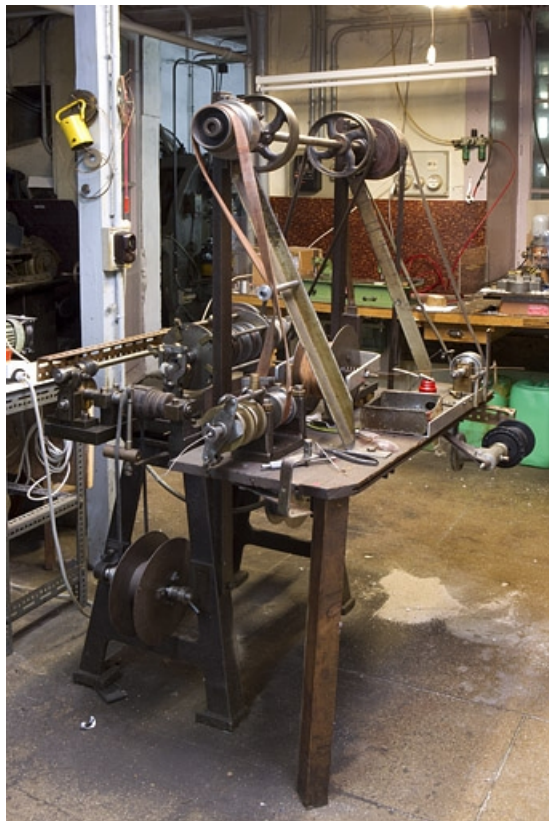
Vue d'ensemble de la face arrière, de trois quarts gauche. Le module de cordage avec les fils de nickel est au centre, avec à gauche celui de cordage avec fils de cuivre et à droite, au deuxième plan, celui du bobinage.
