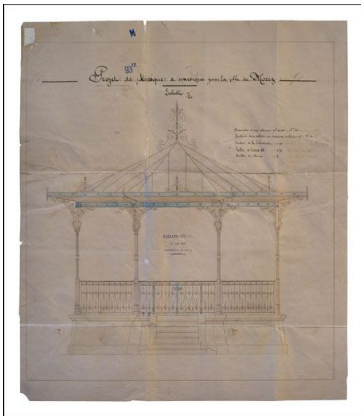
Projet de kiosque à musique pour la ville de Morez, 1899.
