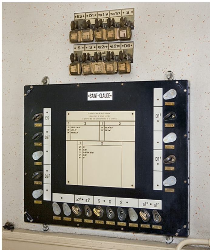
Vue d'ensemble, de trois quarts droite. Cadenas et clefs de secours sont stockés au-dessus de la serrure centrale. 39, Saint-Claude place de la Gare
