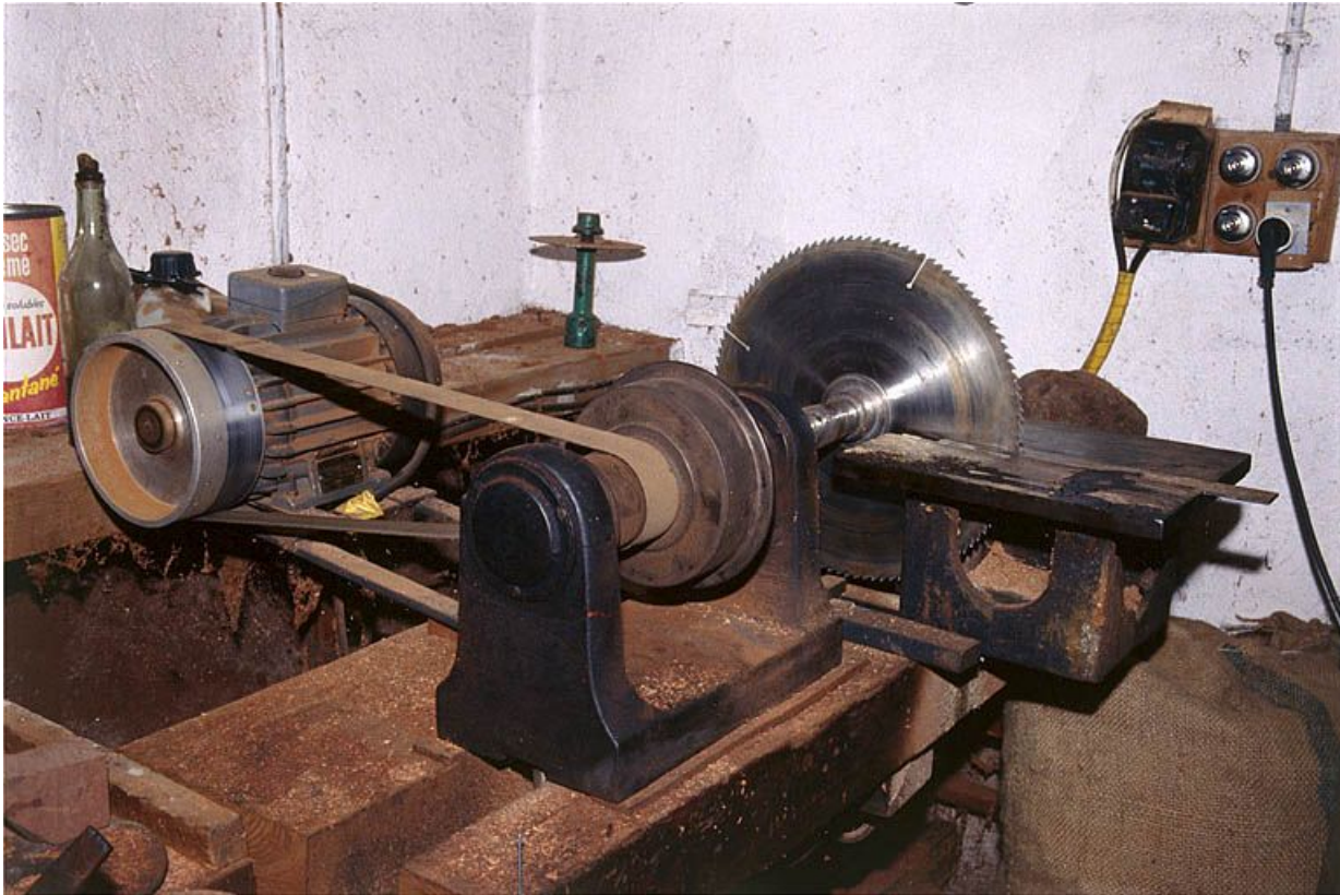
Vue d'ensemble de la scie de droite, servant au franchissage (mise à longueur).
