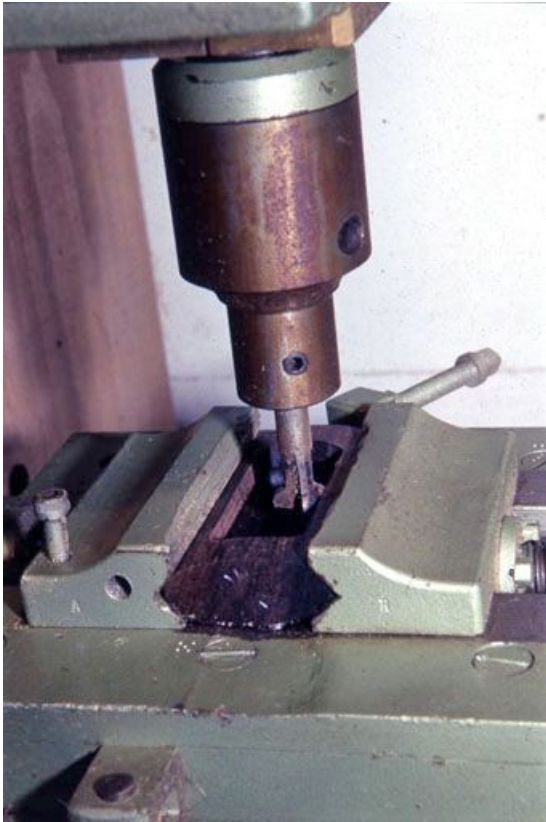
Détail de la fraise.
