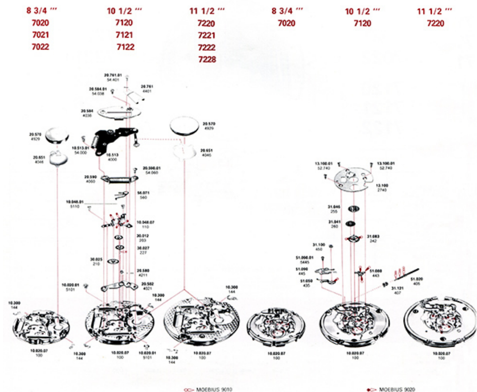
[Vue éclatée des mouvements FE 7020 7021 7022 7120 7121 7122 7220 7221 7222 7228], 1988. 25, Villers-le-Lac
