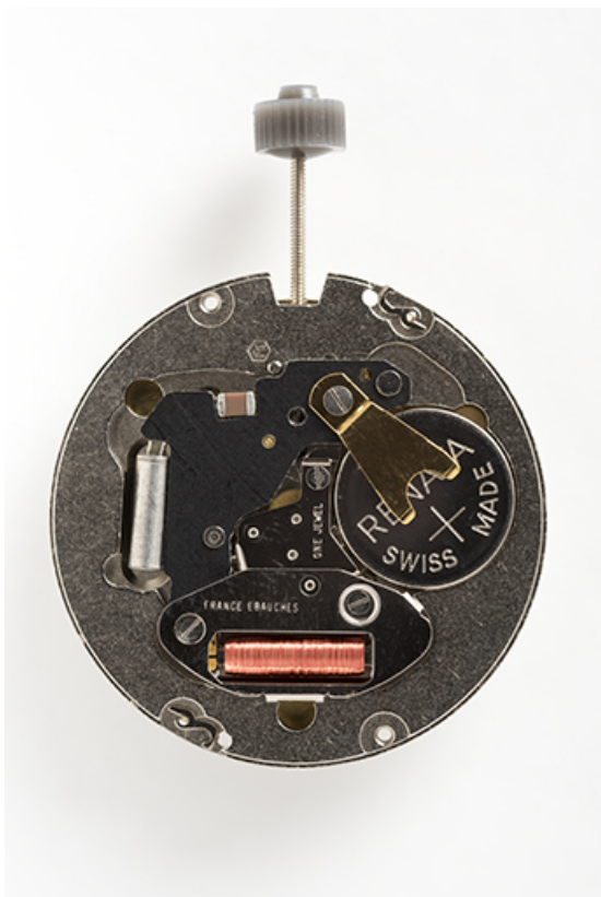
Mouvement France Ebauches FE 7221 : face côté fond. 25, Villers-le-Lac
