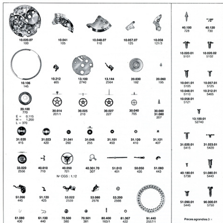
Calibre 11 1/2" 5601 [liste des fournitures], 1980. 25, Villers-le-Lac
