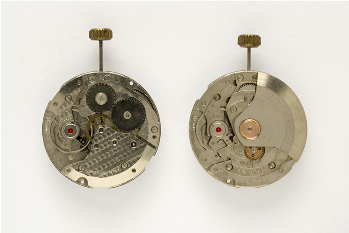
Mouvements France Ebauches FE 5601 (à gauche) et FE 5611 (à droite) : face côté ponts. 25, Villers-le-Lac
