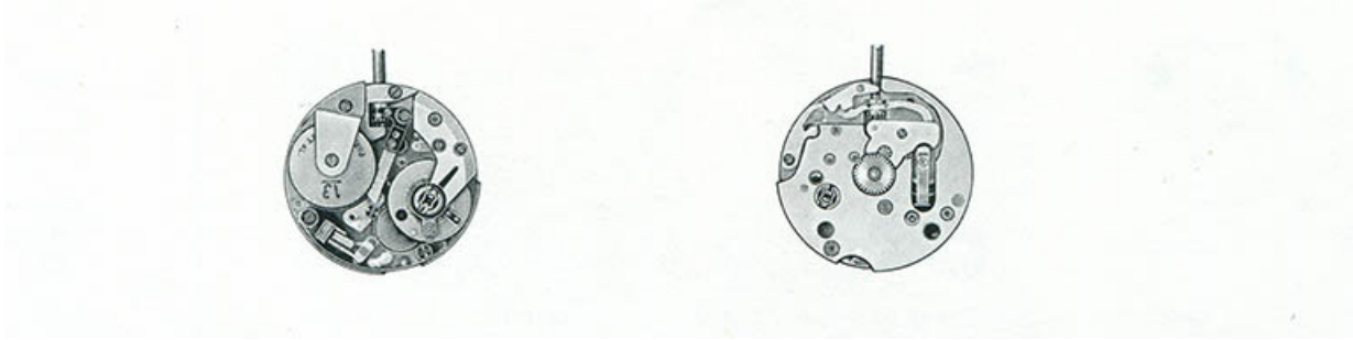
[Dessin du mouvement Lip RE 50], 1973. 25, Maîche
