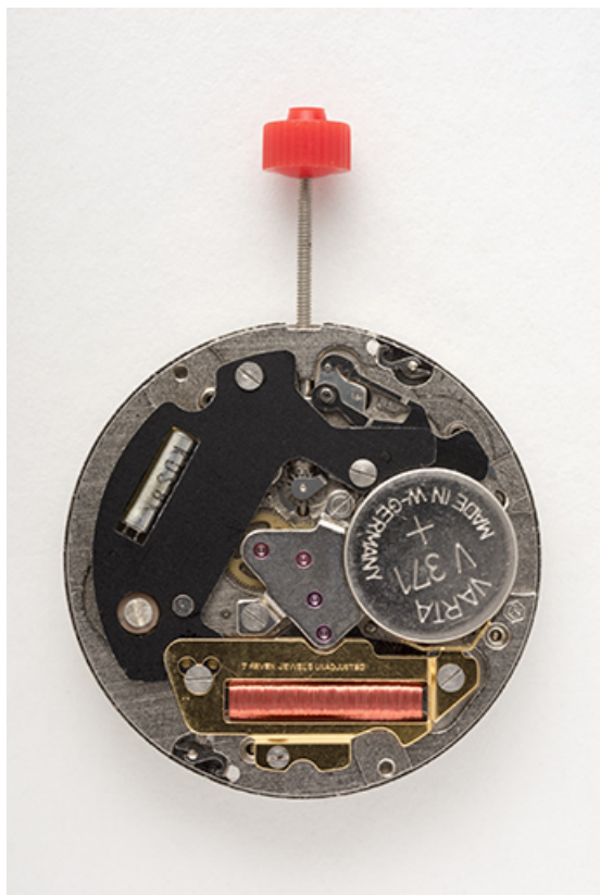
Mouvement FE 11500, vu côté ponts. 25, Maîche
