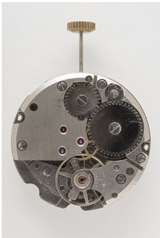
Mouvement FE 140-2A, vu côté pont. 25, Maîche
