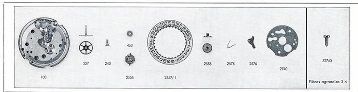
Calibre 11 \frac{1}{2} ''' - 140-1 - Calendrier - (fournitures particulières), 1973.
