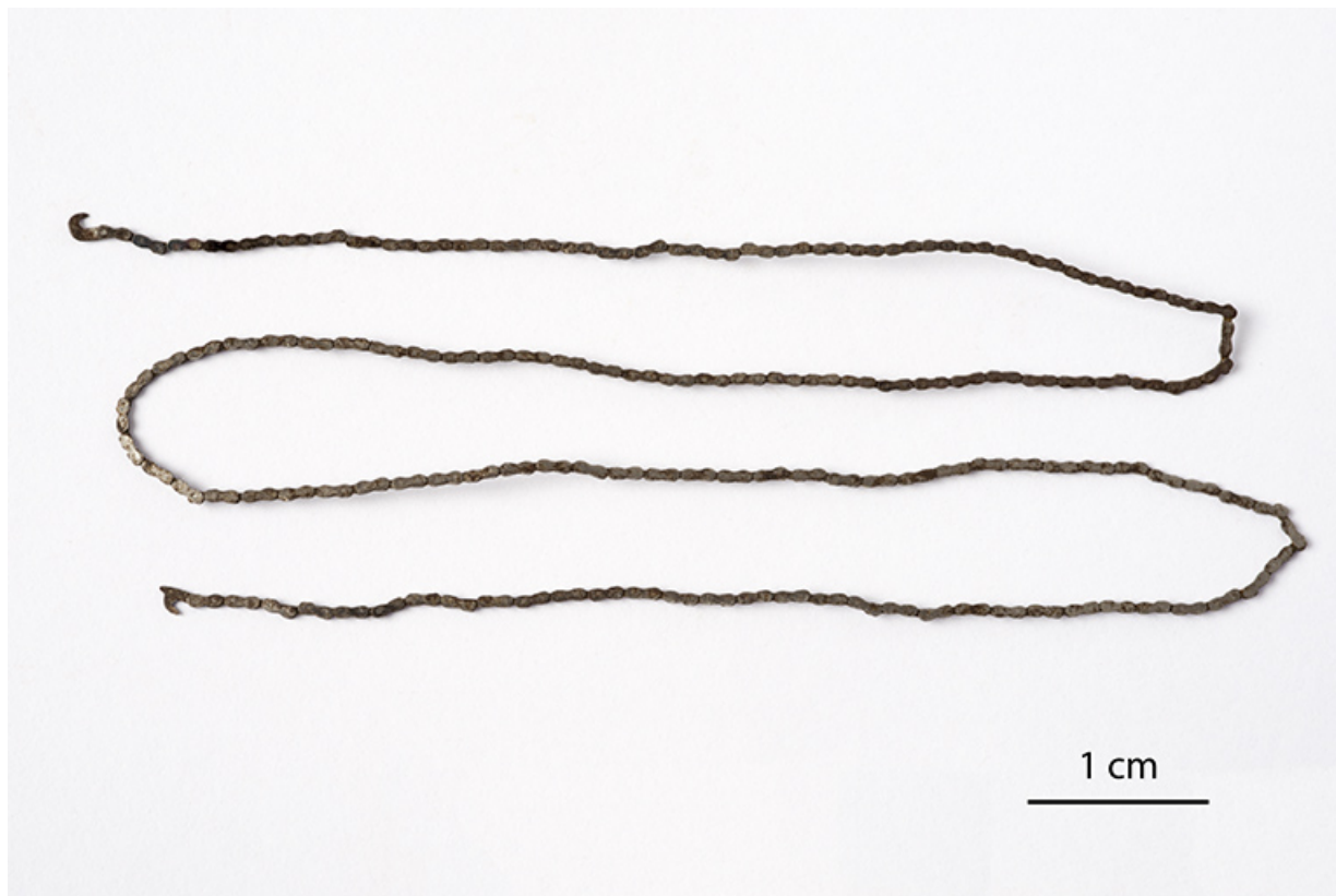
Chaîne de fusée en acier (27 cm de long). Ce type de chaîne était fabriqué à domicile, plutôt par des femmes. 25, Charquemont, 12 Rue Neuve
