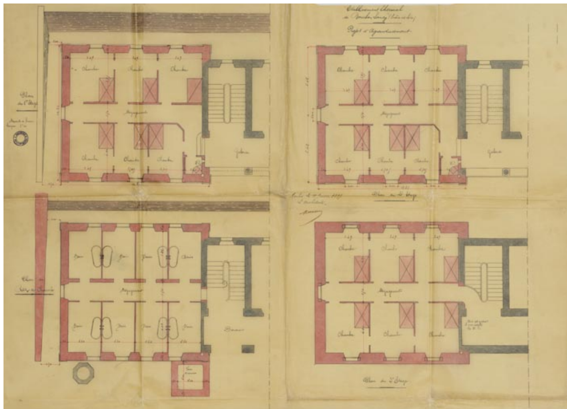
Projet de pavillon annexe, par l'architecte René Moreau (11 janvier 1897), plan des différents niveaux. 71, Bourbon-Lancy, 2 Parc thermal
