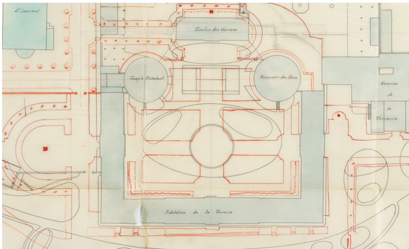
Habitation de la Verrerie. Projet de transformation des abords. N° I [détail]. 21 janvier 1904. 71, Le Creusot rue Jules Guesde
