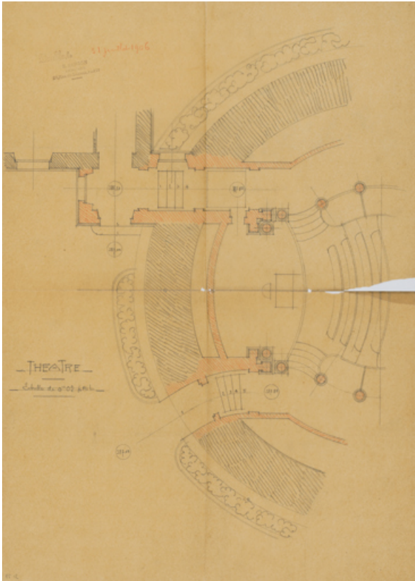
Théâtre [détail des accès]. 31 juillet 1906.
