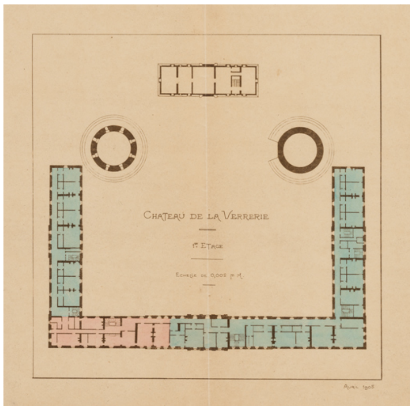
Château de la Verrerie. 1er étage. Avril 1905.
