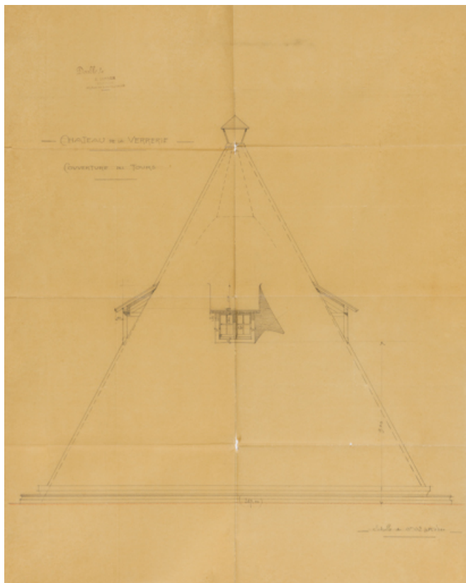
Château de la Verrerie. Couverture des tours. S.d. [1906 ?].
