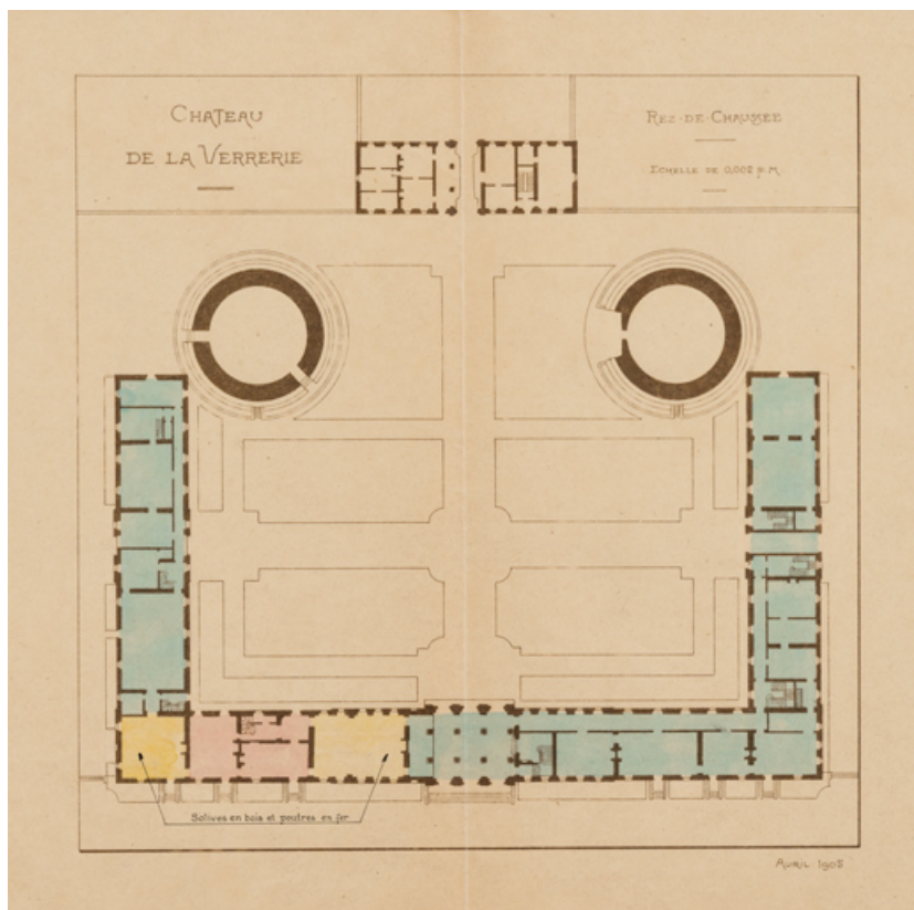
Château de la Verrerie. Rez-de-chaussée. Avril 1905.
