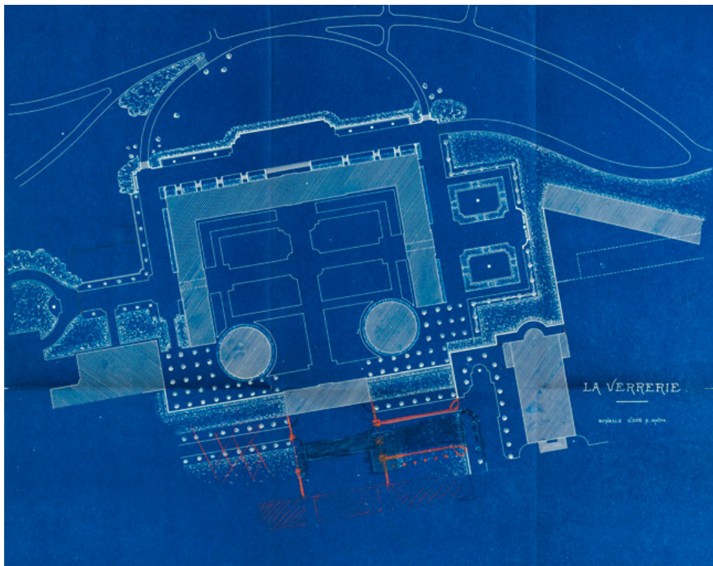
La Verrerie [plan-masse et de situation]. S.d. [1905].
