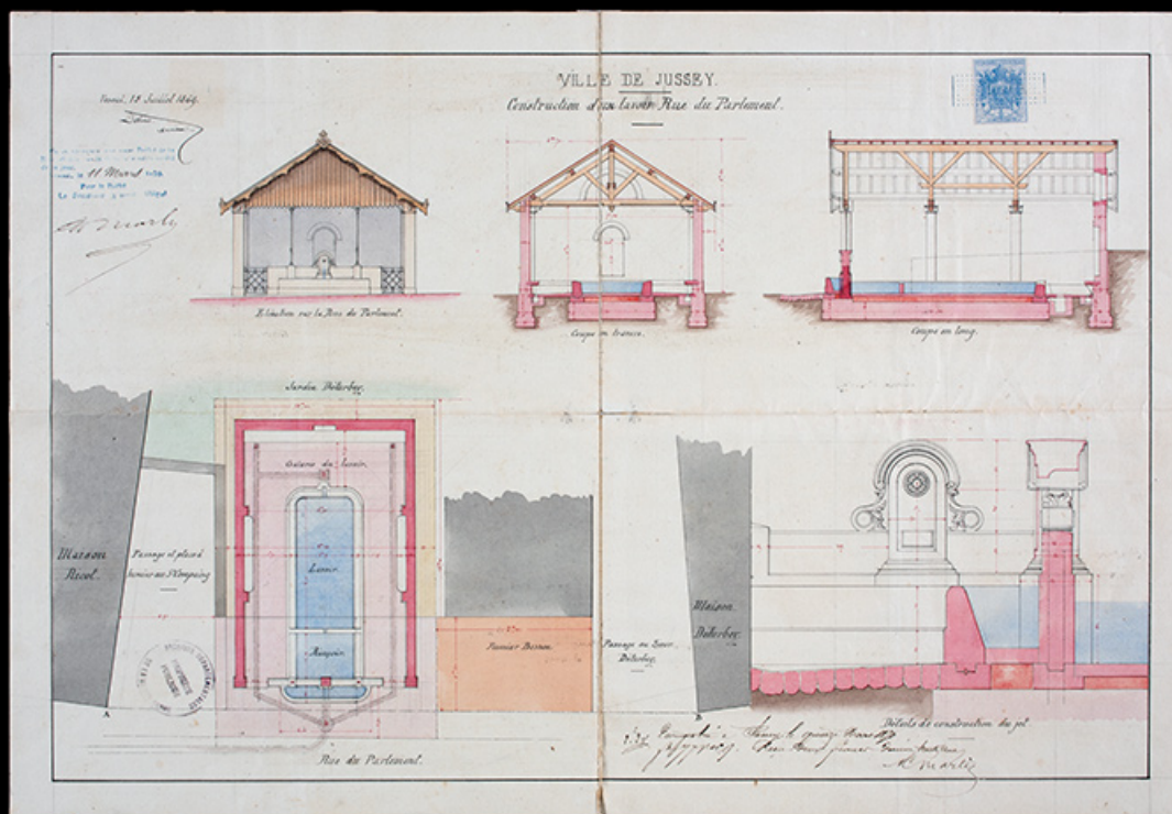
Plan, élévations, coupes et vue de détail de la fontaine-lavoir rue du Parlement à Jussey, 1869.
