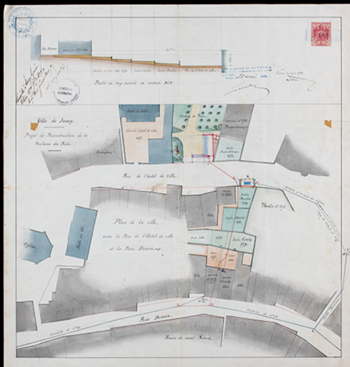
Plan projeté de l'adduction en eau de la fontaine-lavoir des Rois de jussey, 30 avril 1870.
