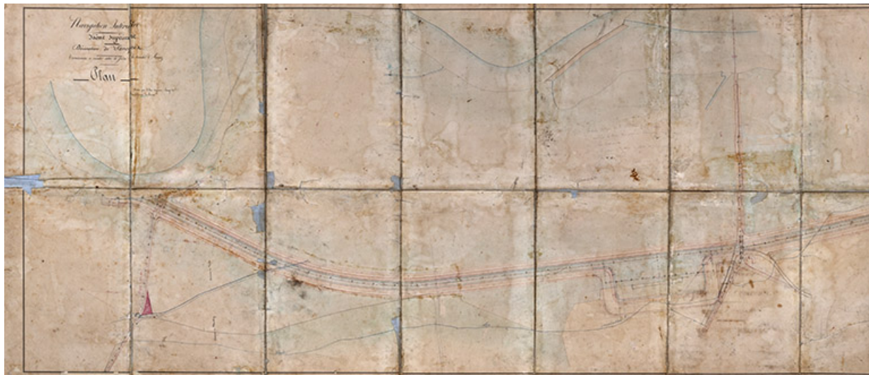
Navigation intérieure, Saône supérieure, dérivation de Savoyeux - Terrassements à exécuter entre la Saône et la partie amont de l'entrée du souterrain [s.d].
