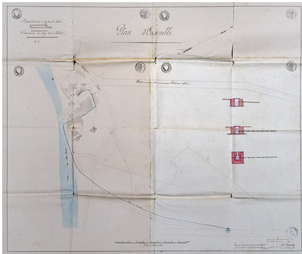
Ringuet. Plan d'ensemble [de la conduite de la source Javelet]. 1841.
