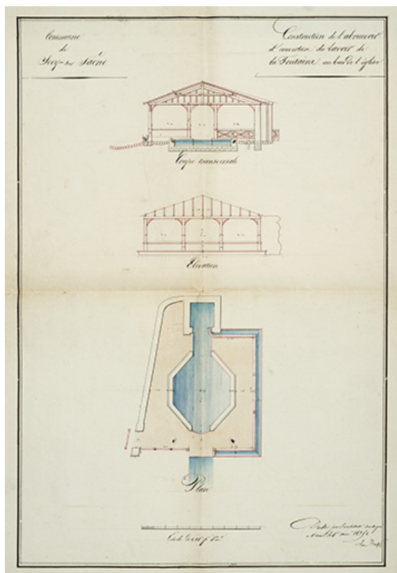
Le Beuffe. Construction de l'abreuvoir et couverture du lavoir de la fontaine au bas de l'église. 1835.
