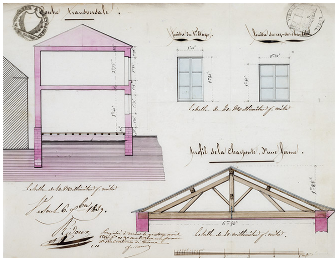
Plan en coupe de la maison commune et détails des fenêtres et de la charpente, 1839 70, Baulay rue de l' Église
